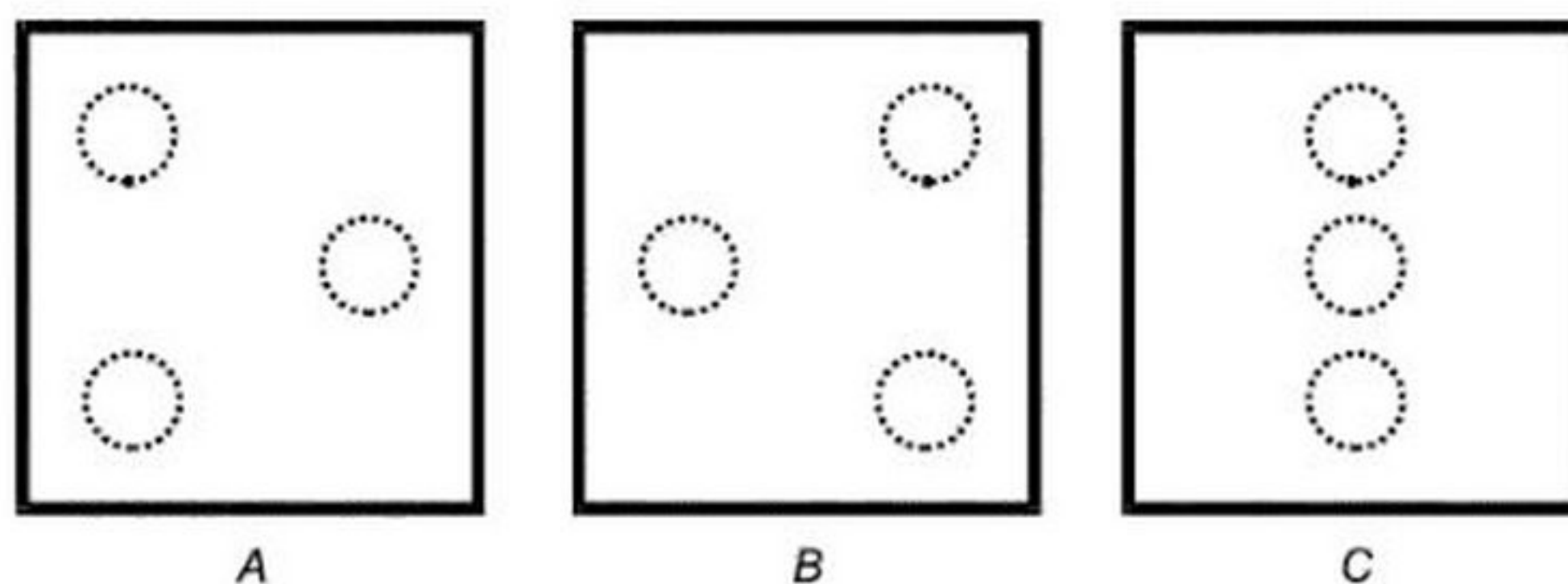
б) Зоны ударов при испытании шариками (для каждого типа остекления)
