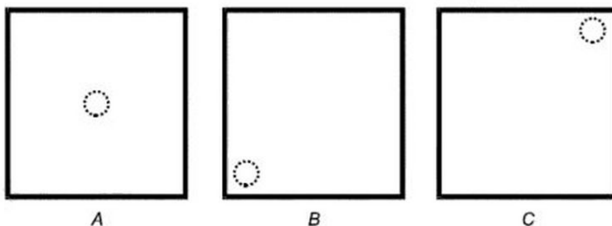
а) Зона удара при испытании деревянным снарядом (для каждого типа остекления)
