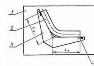
1-контрольная плита; 2- изделие; 3-шаблон; 4- поле допуска
