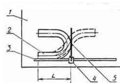
1- контрольная плита; 2-изделие; 3- контрольная линейка; 4- ползун; 5-упор
