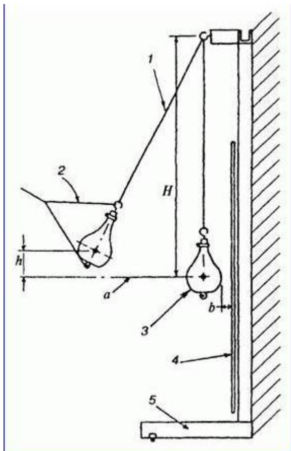
1-стальной трос диаметром 2,5-4 мм; 2-уздечка для подъема мешка; 3-кожаный мешок (мягкое тело); 4-испытываемый образец, закрепленный в стенде; 5-опора; H -высота подвеса; h -высота падения мешка; a -центральная ось испытываемого образца; b -расстояние между образцом и мешком, висящим в свободном состоянии
